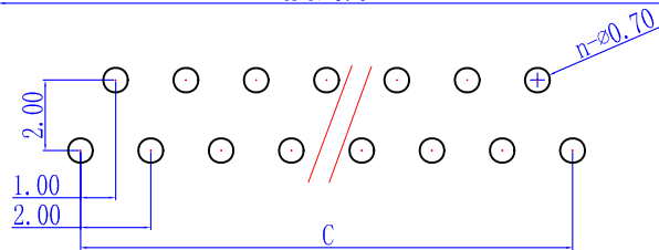
1.0-B2-nPW 印制线路板 P.C.B Layout
